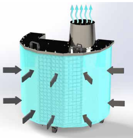
Luftführung ohne Leitblech
