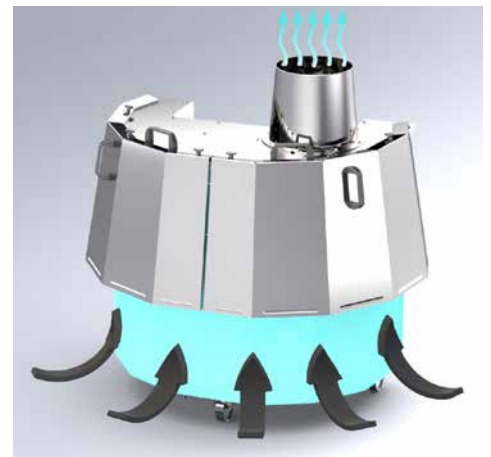
Luftführung mit Leitblech (optional)
